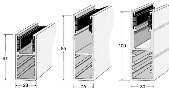
Styrskenor HSF, HST-F och SHST-F
