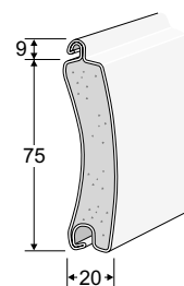
Lamellprofil 75 D
