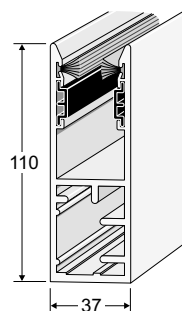
Styrskena URF 110
