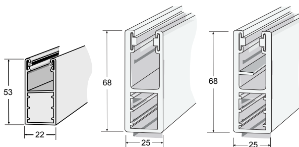
Styrskenor HTF, Safe N och Safe S
